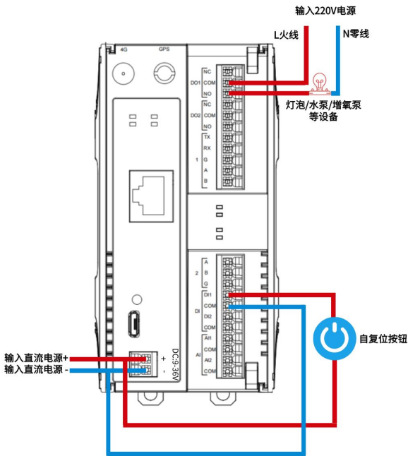
(1) 【手动控制开关接线图】
